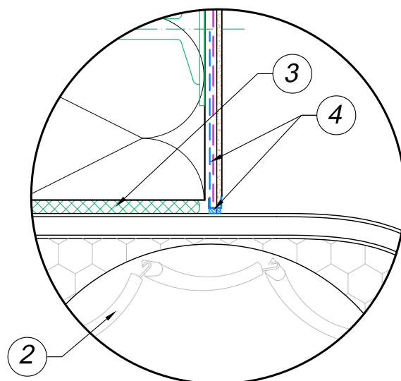
Nr. 1.3.11 Ocieplenie nadproża z żaluzją okienną zewnętrzną
