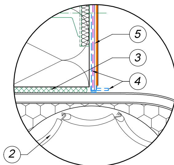
Nr 1.3.9. Ocieplenie nadproża z żaluzją okienną zewnętrzną
