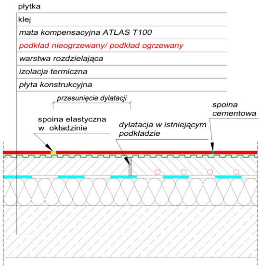
Rys. 1 Rozwiązanie tradycyjne - płytki ceramiczne ułożone na podkładzie z ogrzewaniem podłogowym i bez ogrzewania. Dylatacja w podłożu przeniesiona na posadzkę z płytek ceramicznych.
